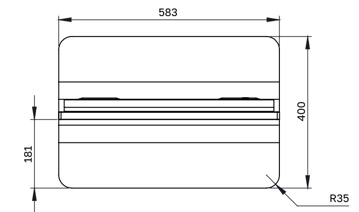
СХЕМА ДИСПЛЕЯ (ВИД СВЕРХУ)
